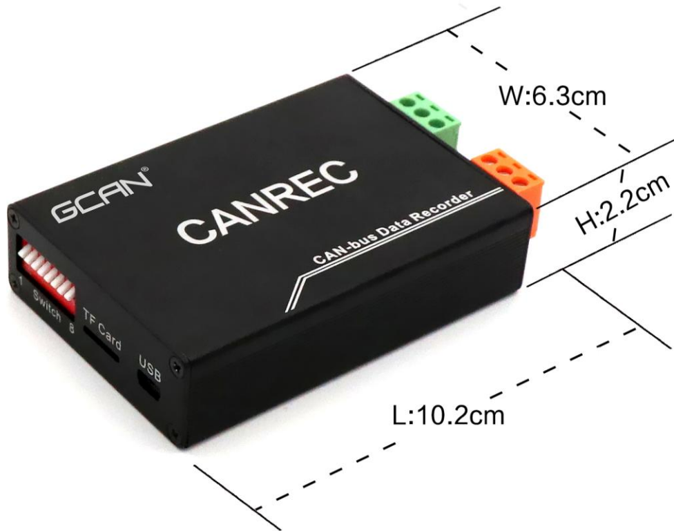
图 2.1 GCAN-401 外形尺寸
