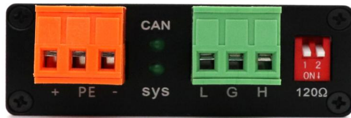
图 2.2 GCAN-401 模块电源端子接口
